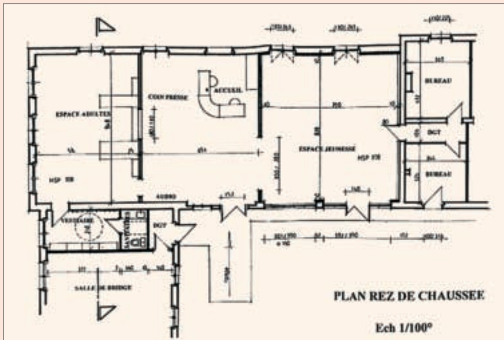
Le plan de l'extension de la bibliothèque
